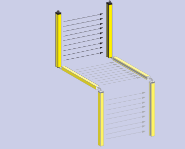
GuardShield (PAC)-Sicherheitslichtgitter (Zugangsabsicherung)
